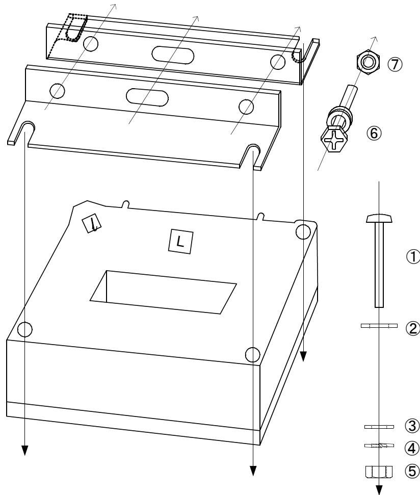
使用部品表
